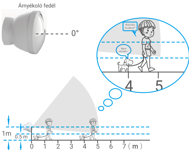
1. ábra Az érzékelési tartomány oldalnézete
