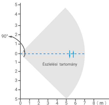
2. ábra Az érzékelési tartomány felülnézete
