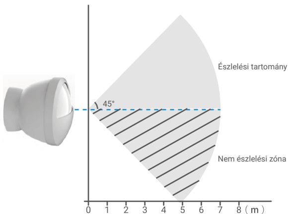
2. ábra Az érzékelési tartomány felülnézete
